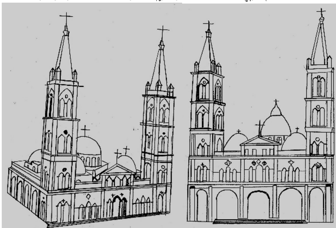
شكل ٤ الواجهة الغربية القديمة قبل الزيادة لكنيسة السيدة العذراء مريم بالأقصصر والتي ترجع للربع الأخير من القرن ١٩م عمل الباحث © تنشر لأول مرة
