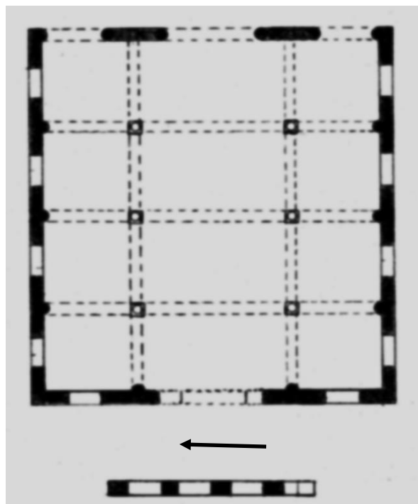
شكل ٣ القسم الغربي من كنيسة السيدة العذراء مريم بالأقصصر عمل الباحث © تنشر لأول مرة
