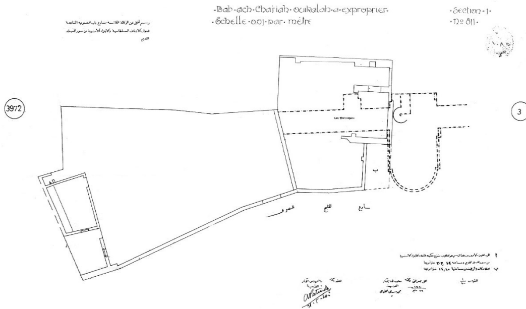
(شكل 6) مسقط أفقي لبقايا باب القنطرة والجزء الشمالي من سور القاهرة الغربي عن رسومات مركز تسجيل الآثار
